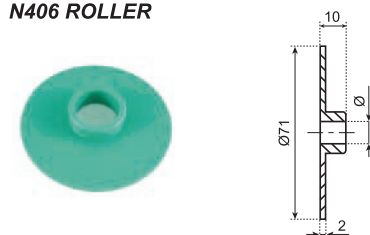
N406 托轮 N406 ROLLER
