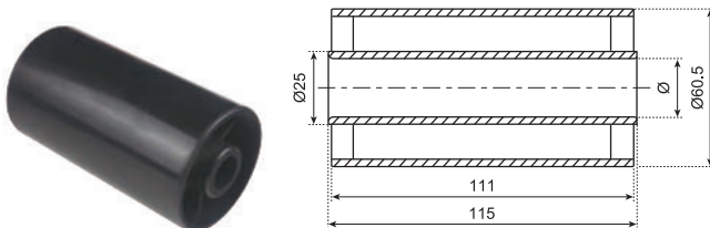
N421 托轮 N421 ROLLER
