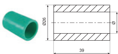
N413 托轮 N413 ROLLER
