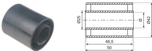
N419 托轮 N419 ROLLER
