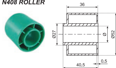
N408 托轮 N408 ROLLER
