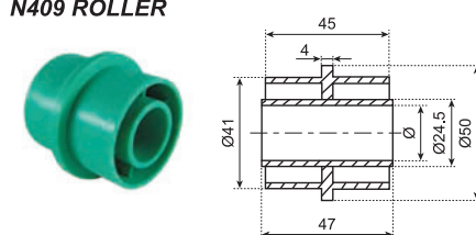
N409 托轮 N409 ROLLER
