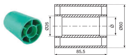
N405 托轮 N405 ROLLER
